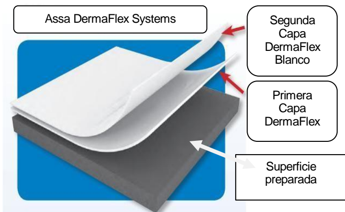
Sobre techo limpio existente o resellado
